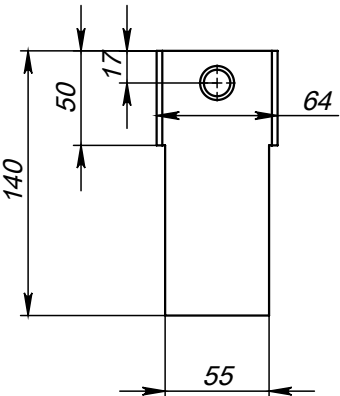
Поз.4 (Пластина)
