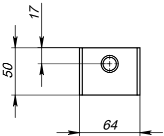
Поз.3 (Пластина)
